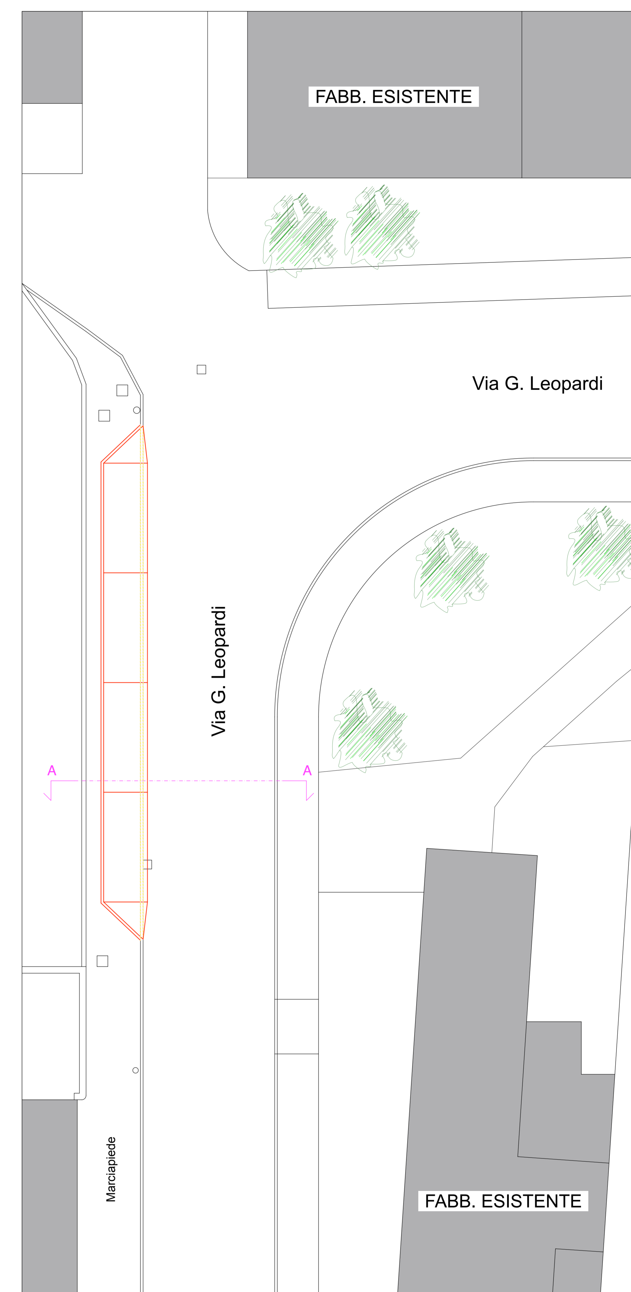
PLANIMETRIA DI SOVRAPPOSIZIONE scala 1:100
