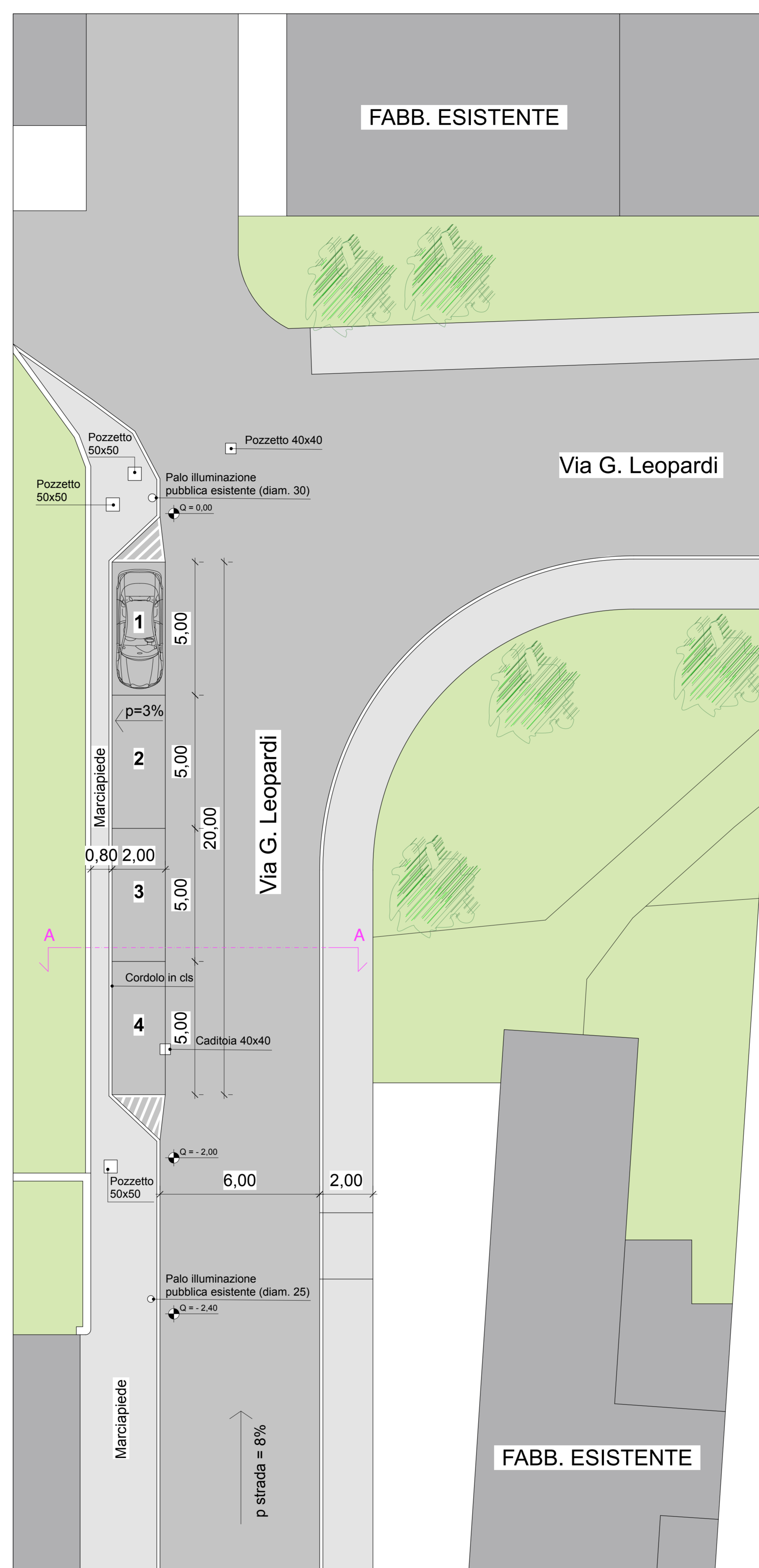
PLANIMETRIA DI PROGETTO scala 1:100
