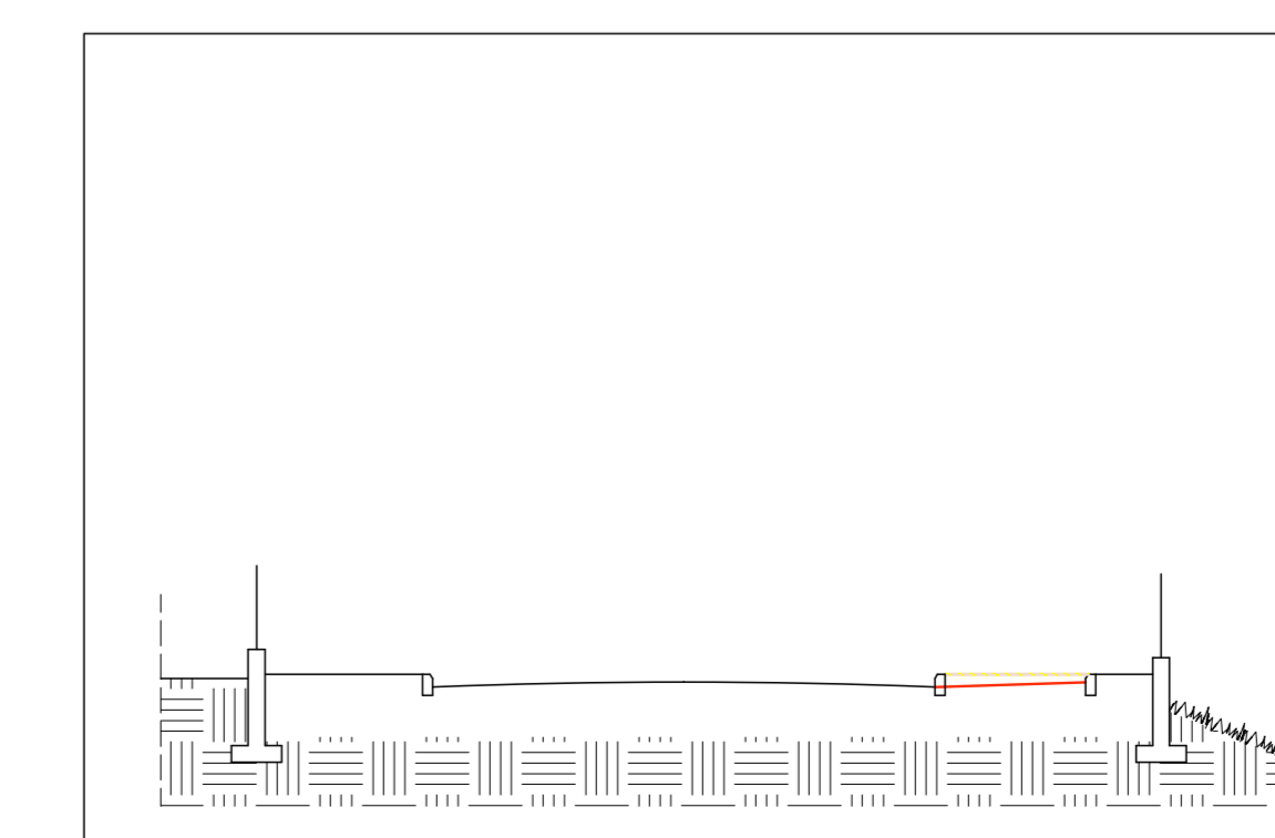
SEZIONE DI SOVRAPPOSIZIONE scala 1:100
