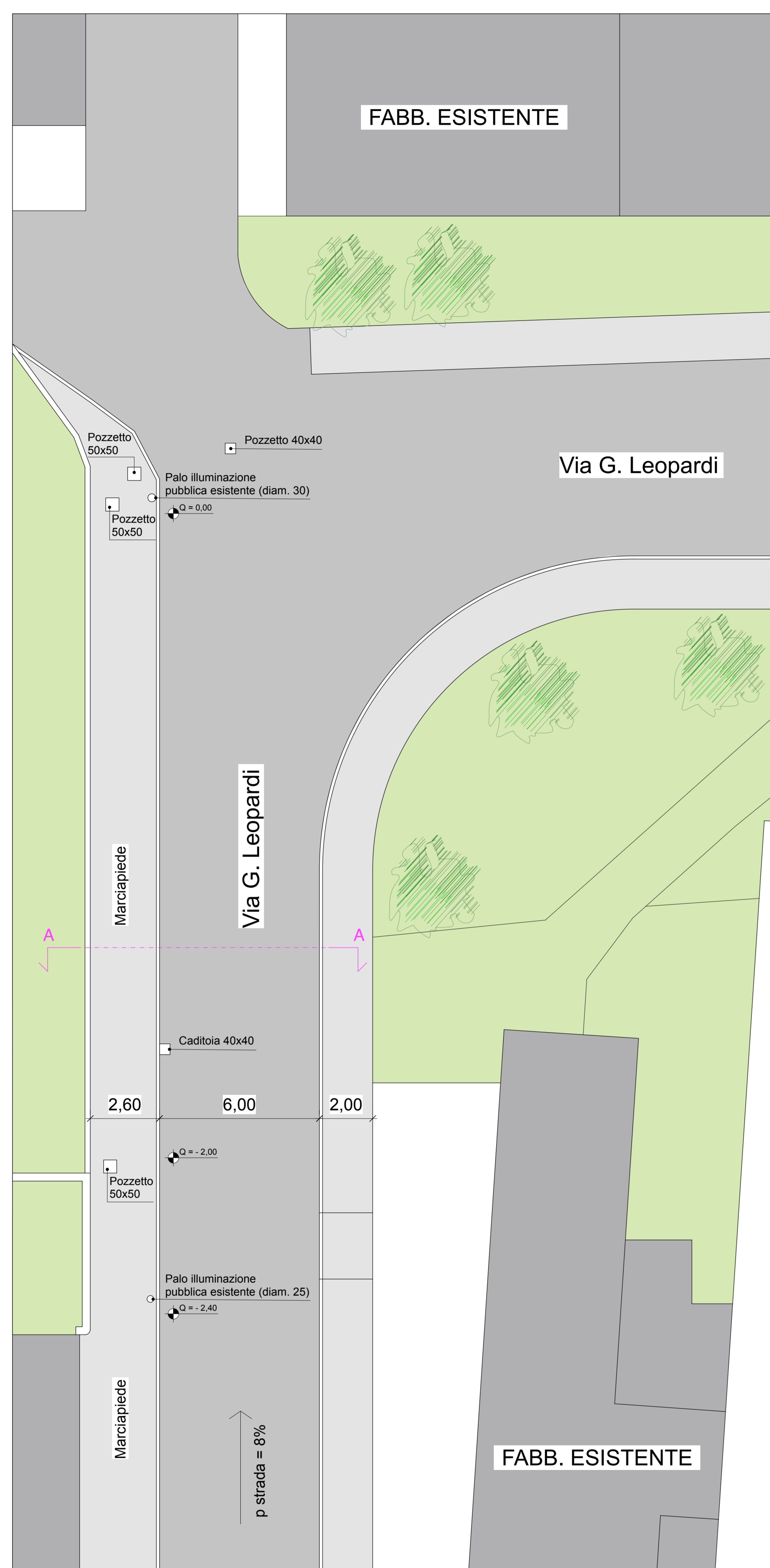
PLANIMETRIA STATO DI FATTO scala 1:100
