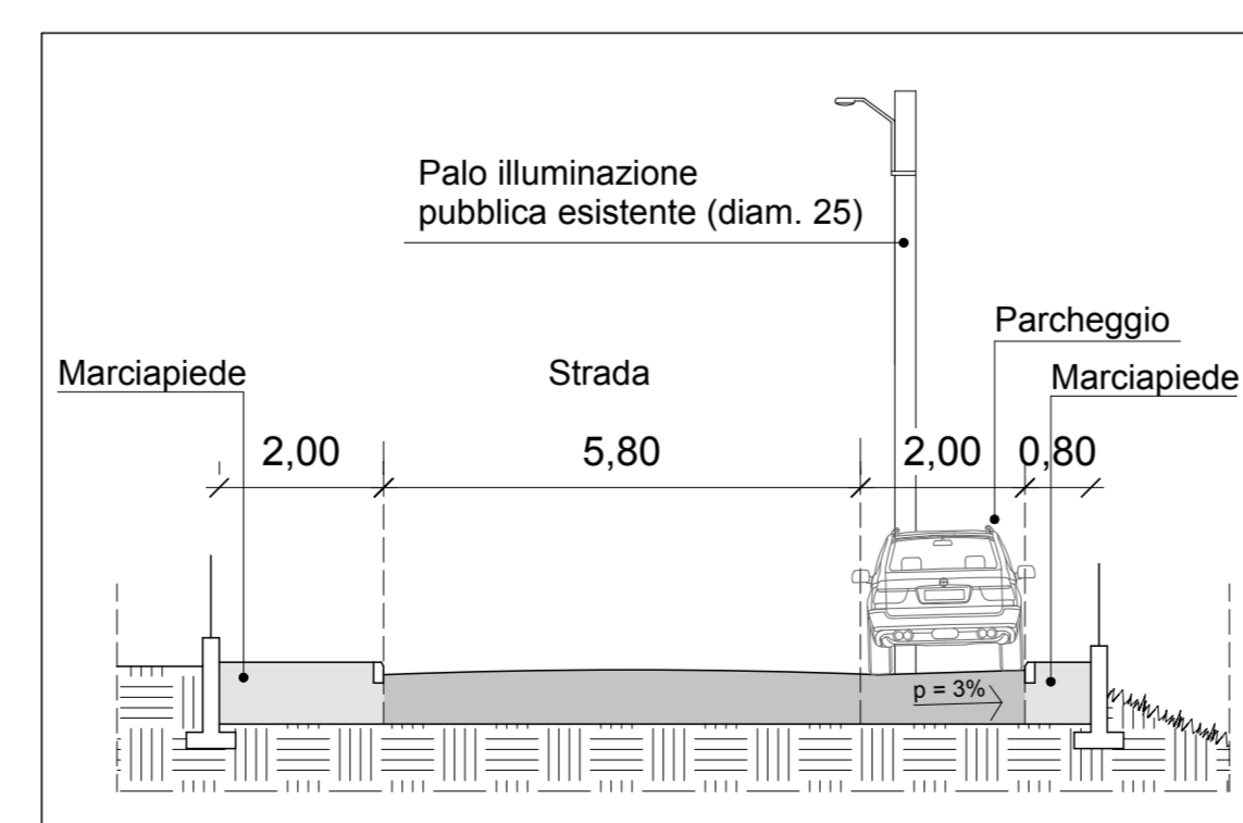
SEZIONE DI PROGETTO scala 1:100
