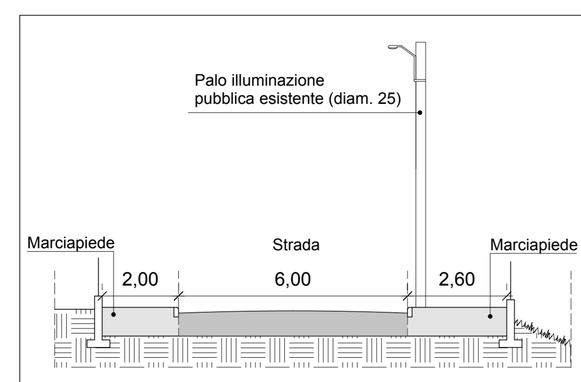
SEZIONE STATO DI FATTO scala 1:100
